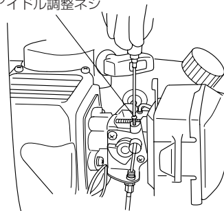
アイドル調整ネジ
