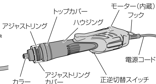
WT 3GP/WT 4GP/WT 5GP (レバーなし)
