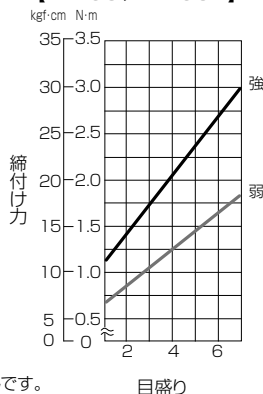
【WT 5G、WT 5GP】
