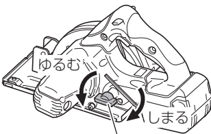
切込み調整用 ちょうボルト
