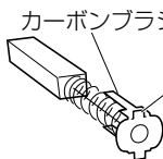
カーボン ブラシのツバ
