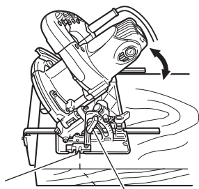
切断位置 (45° の場合) 傾斜用 ちょうボルト
