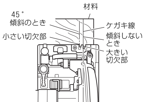
〔上から見た図です〕
