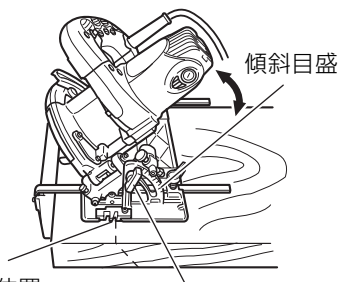
切断位置 (45°の場合) 傾斜用ちょうボルト
