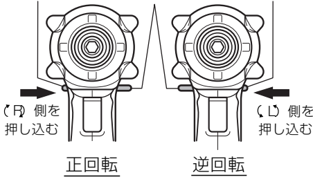
〔工具本体を先端から見た図〕
