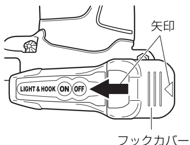
ライト付フック本体
