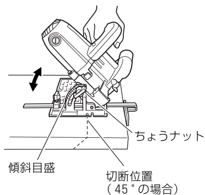
(45° 傾斜のとき)
