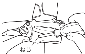
ねじ ライト付フック プラスドライバー (No.1)
