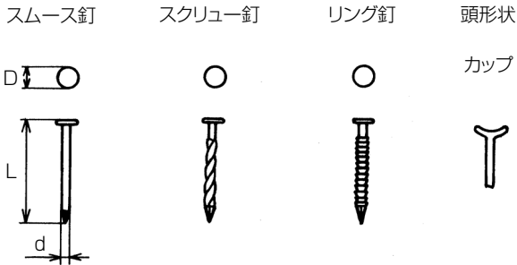
図 3 釘の寸法・形状
