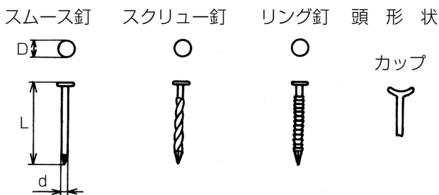
図 3 釘の寸法・形状
