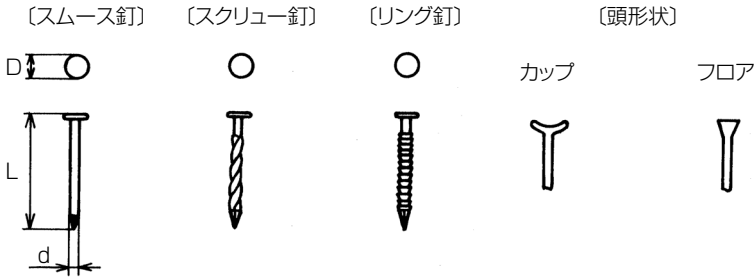
図 3 釘の寸法・形状
