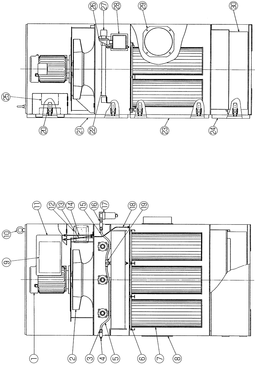
RG 500YA 構造図
