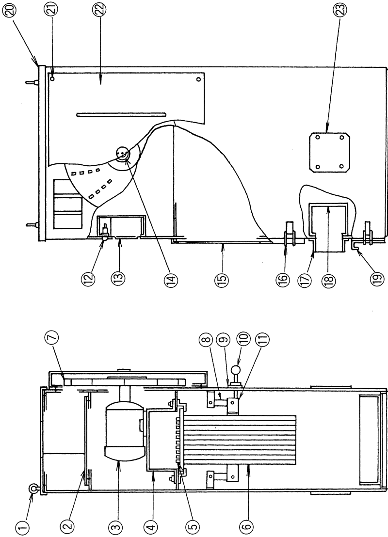
RG 120SA 構造図
