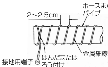
例 1 金属細線によるアース
