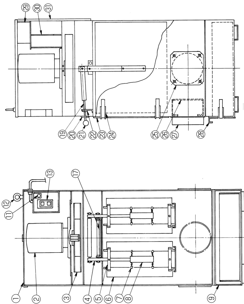
RG 300、RG 500 構造図
