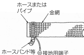
例 2 金網によるアース
