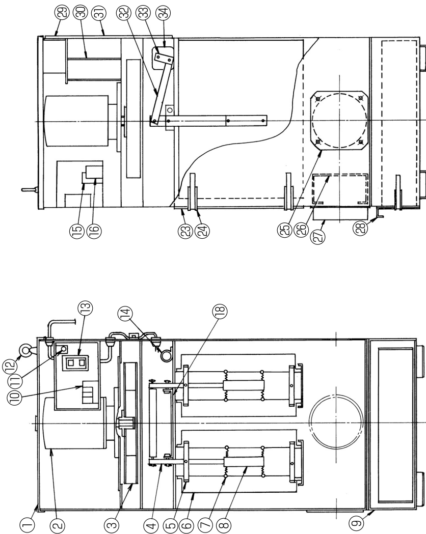
RG 300Y、RG 500Y 構造図 (電動除湿じん形)
