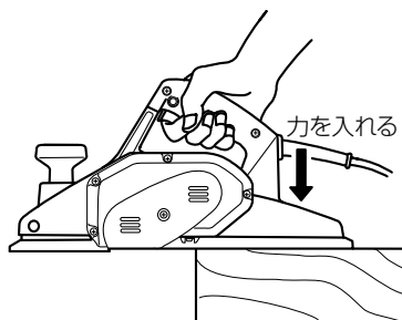
図 9 (削り終り)
