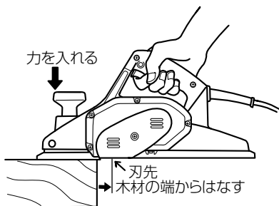
図 8 (削り始め)
