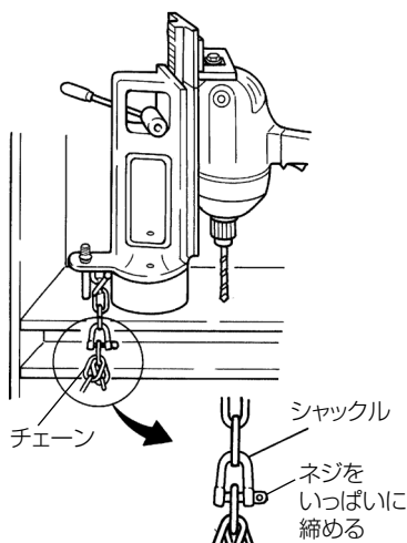
結合部詳細図
