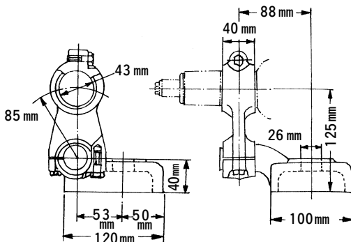
図 7 (寸法図)
